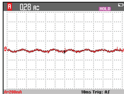
PE current
